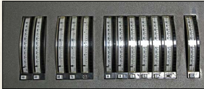
Hauptsteller der Sitralux U. Die Hauptsteller dieser Anlage sind zusammengefasst als Bühne-Vorderhaus, Gruppensteller, Überblender und Intensitätssteller Foto: A. Henrich
